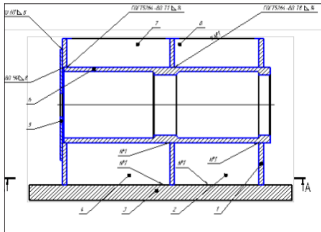
Рисунок 6 – Перевод трехмерной модели в двухмерный чертеж по ЕСКД выполнено программой «Компас 3D V18»
