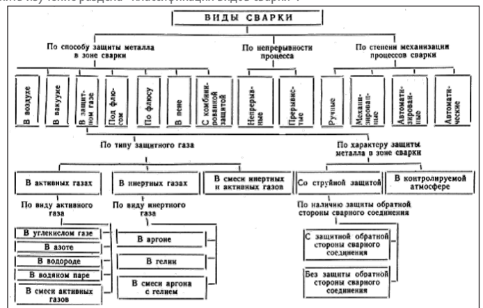
Рисунок 2 – Классификация видов сварки по технологическим признакам
